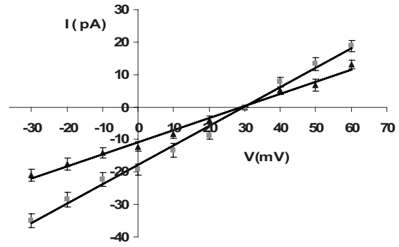
شکل ۲ - منحنی جریان - ولتاژ در محیط 200 mM KCl cis/50 mM KCl trans با subconductance state و مثلث و fully open state با مربع. نقاط بصورت mean \pm SE نمایش داده شده است (n=5)
